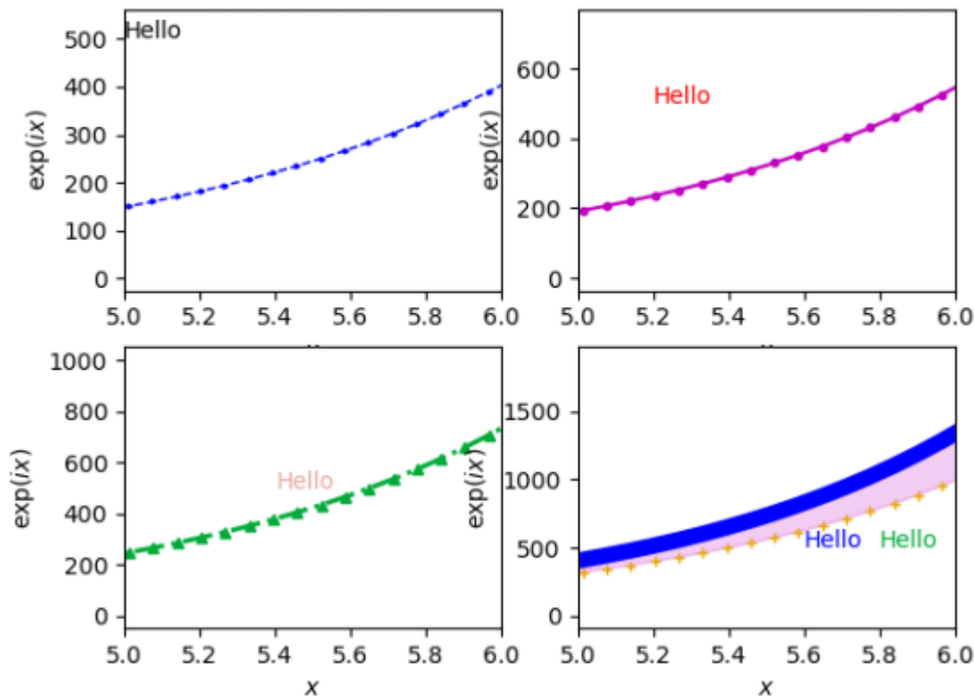
Graphique 2D matplotlib
